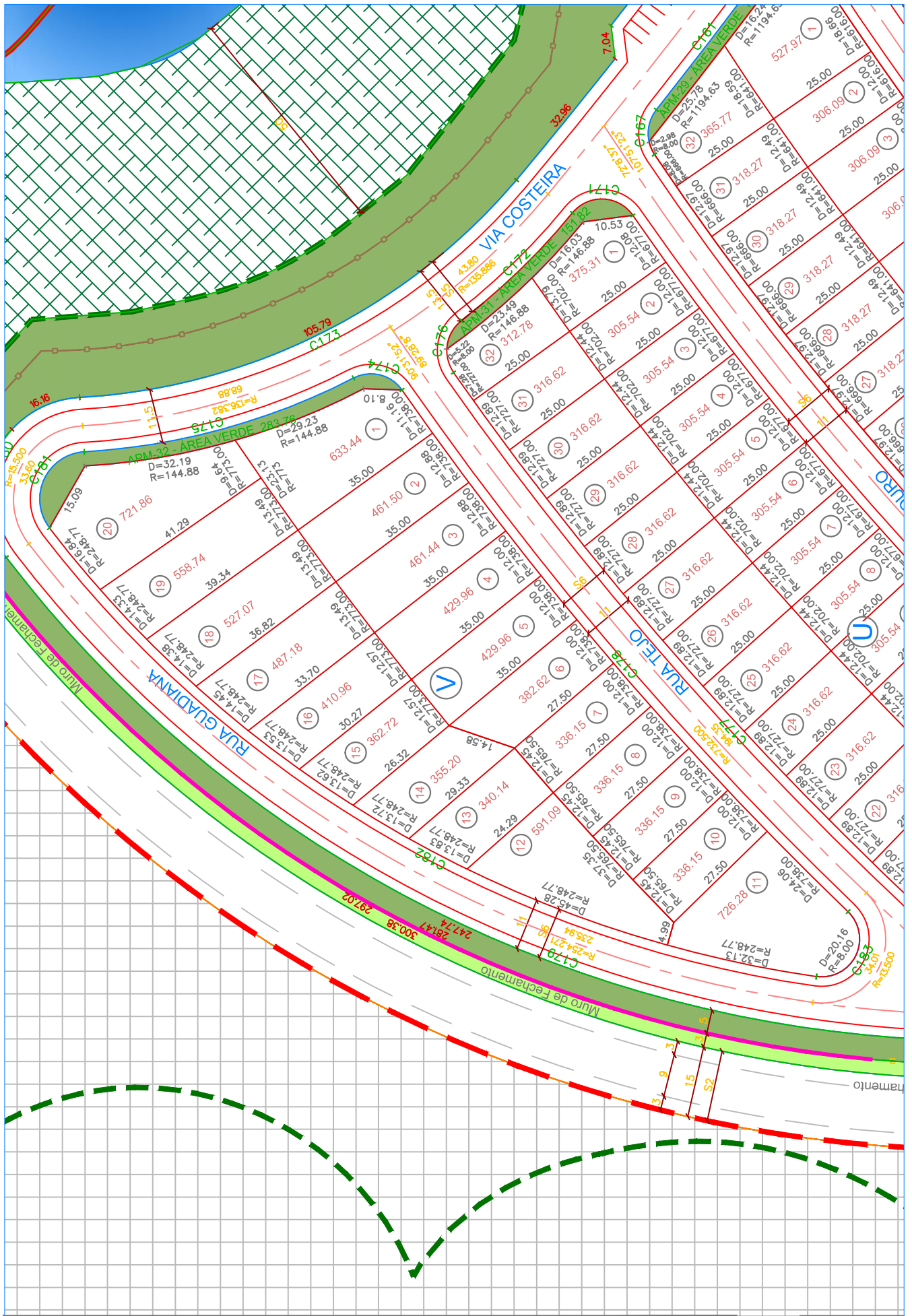
PLANTA DE SITUAÇÃO - QUADRA V
