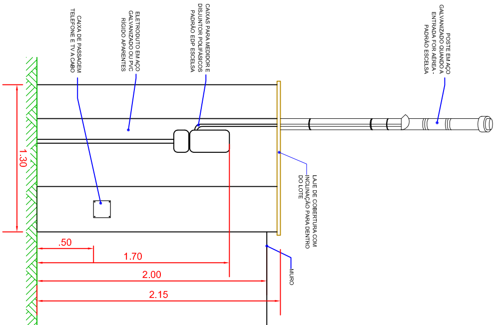
PAREDE DE SERVIÇO - PORTA ABERTA VISTA FRONTAL SEM ESCALA
