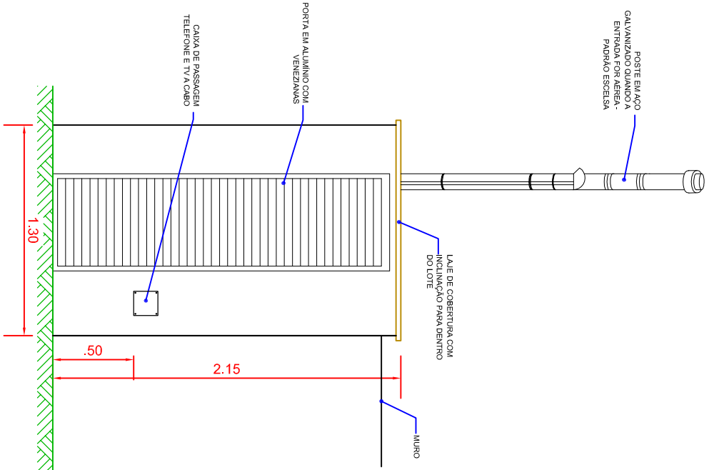
PAREDE DE SERVIÇO VISTA FRONTAL SEM ESCALA
