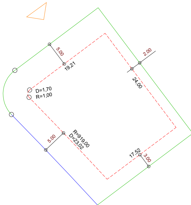
PLANTA DE SITUAÇÃO ESC.: 1/1000
