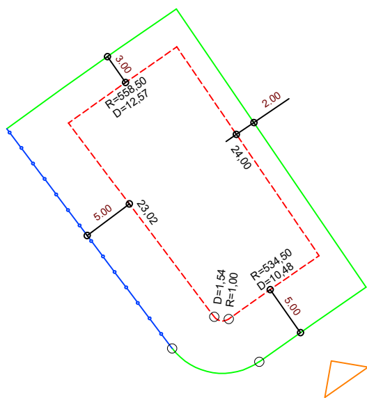
PLANTA DE SITUAÇÃO ESC.: 1/1000
