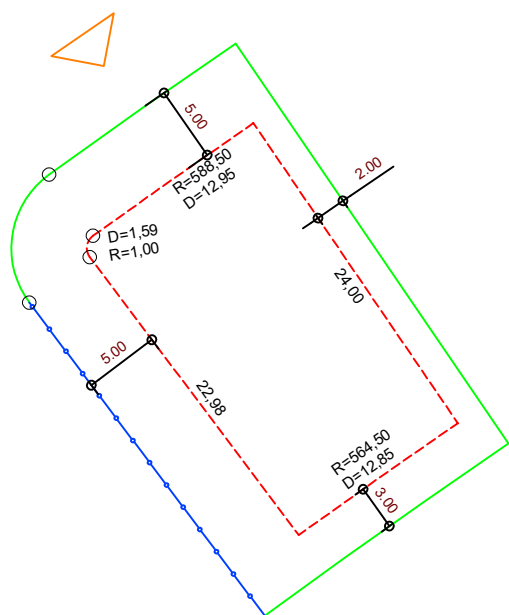
DETALHE DE RECUOS ESC.: 1/500
