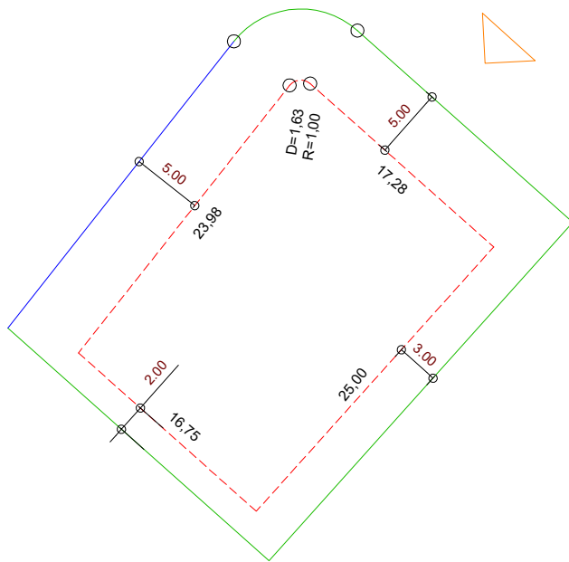
DETALHE DE RECUOS ESC.: 1/500
