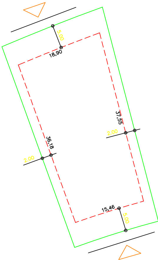
PLANTA DE SITUAÇÃO ESC.: 1/1000
