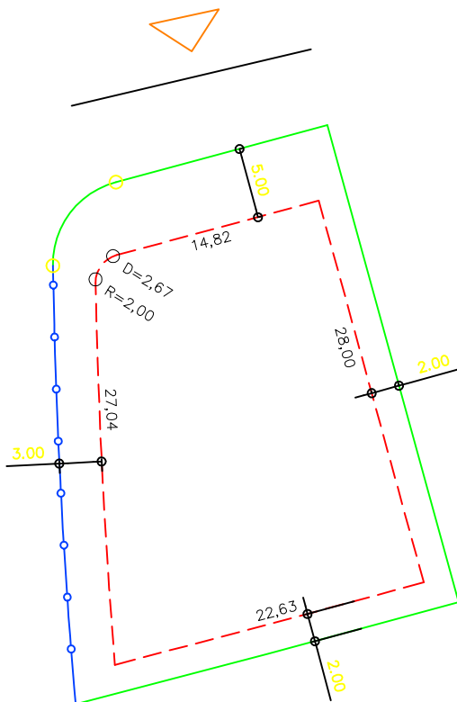
DETALHE DE RECUOS ESC.: 1/500
