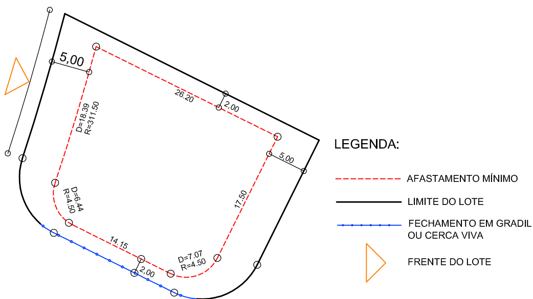
DETALHE DE RECUOS ESC.: 1/500
