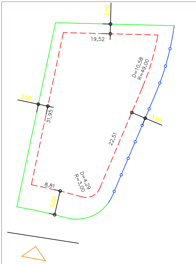
DETALHE DE RECUOS ESC.: 1/500
