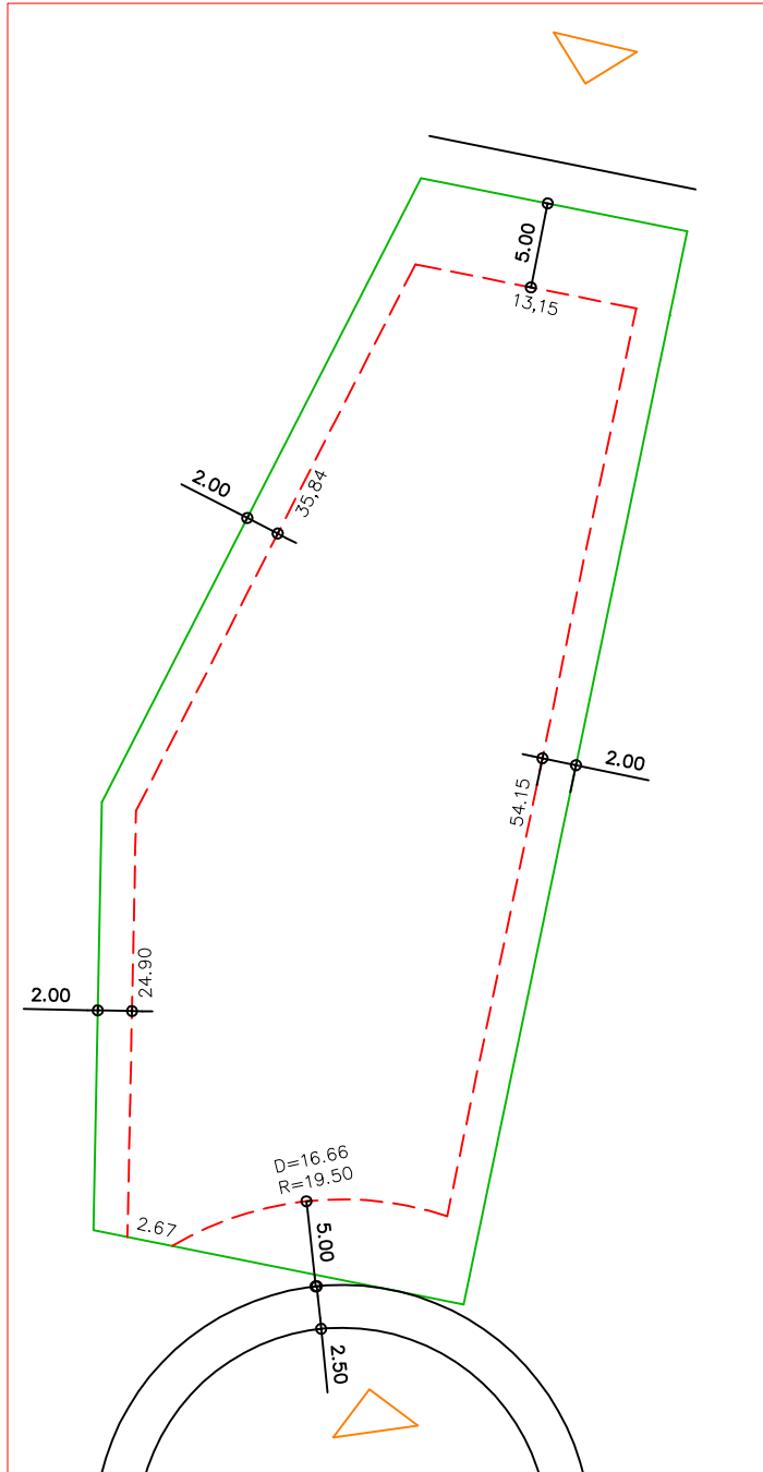
DETALHE DE RECUOS ESC.: 1/500
