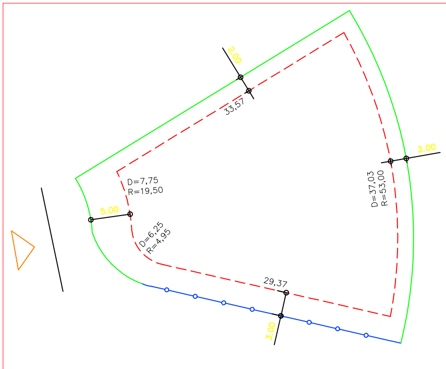
DETALHE DE RECUOS ESC.: 1/500
