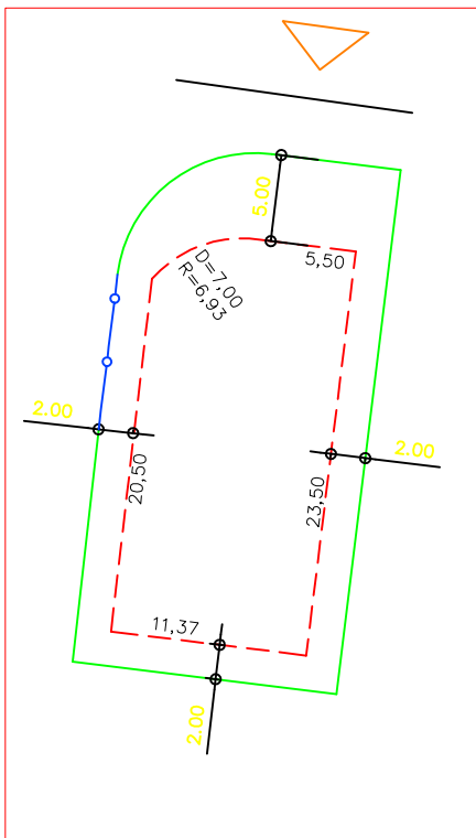
DETALHE DE RECUOS ESC.: 1/500
