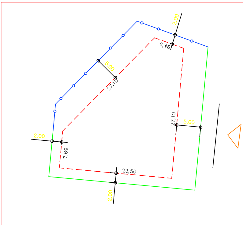
DETALHE DE RECUOS ESC.: 1/500
