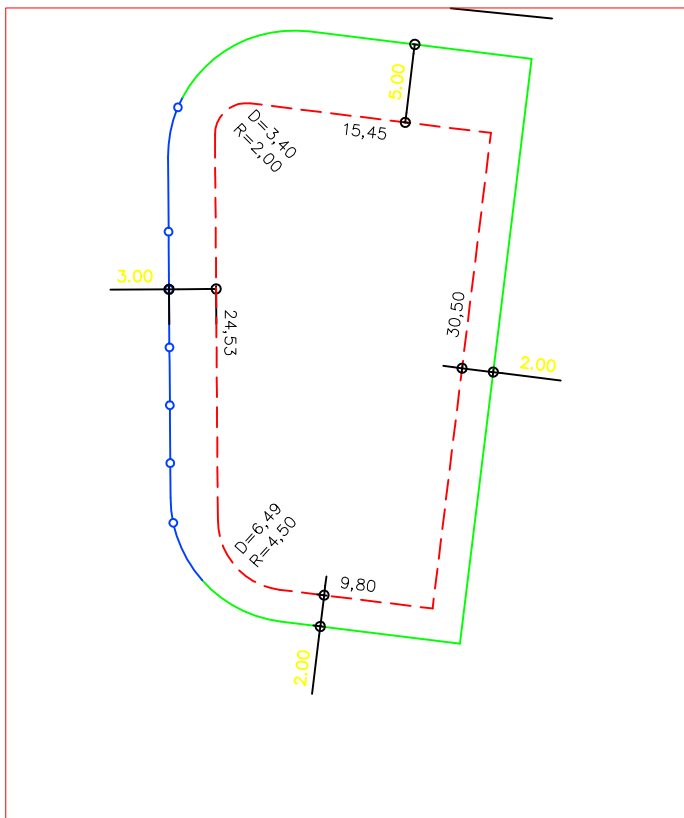
DETALHE DE RECUOS ESC.: 1/500
