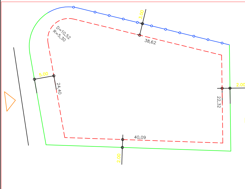
DETALHE DE RECUOS ESC.: 1/500
