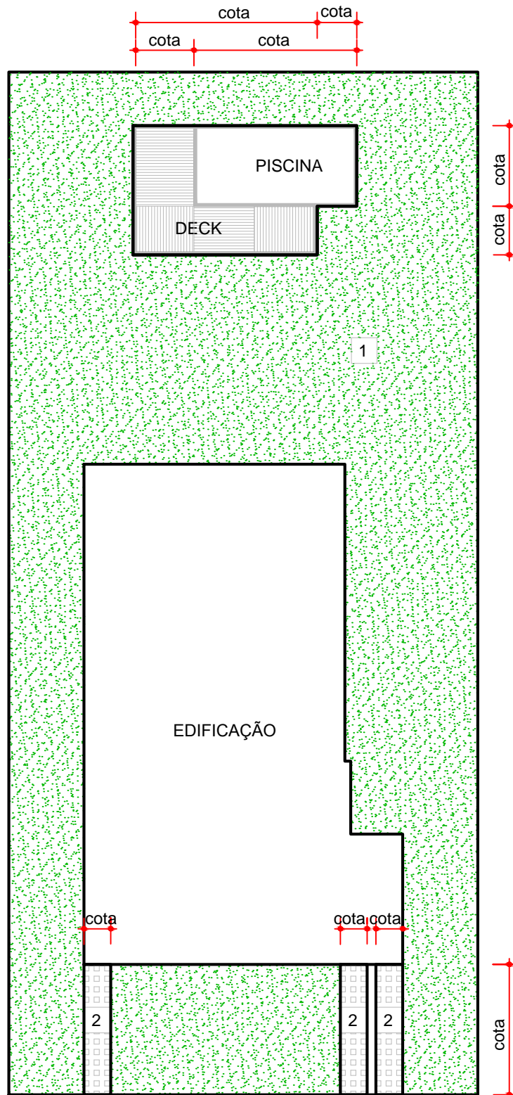
PAVIMENTO TÉRREO Esc. 1:100
