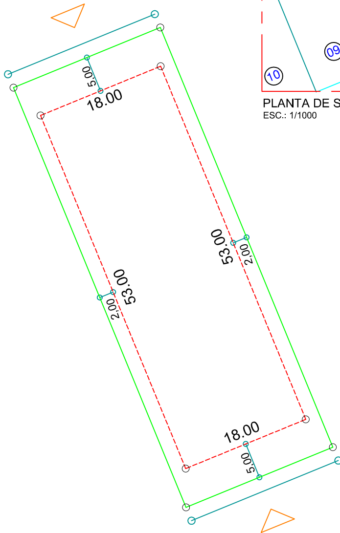
DETALHE DE RECUOS ESC.: 1/500
