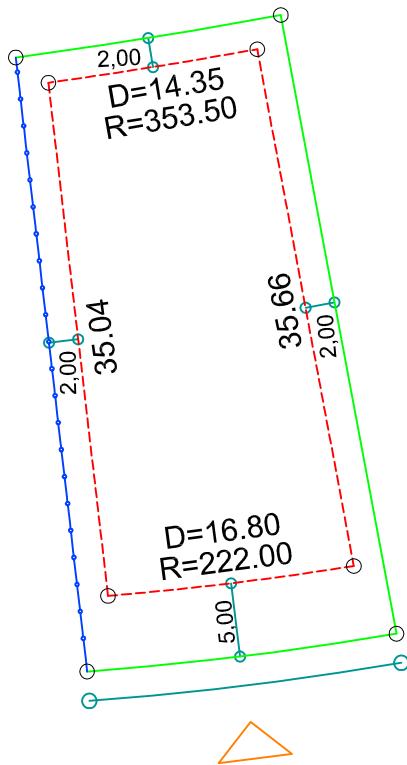
DETALHE DE RECUOS ESC.: 1/500
