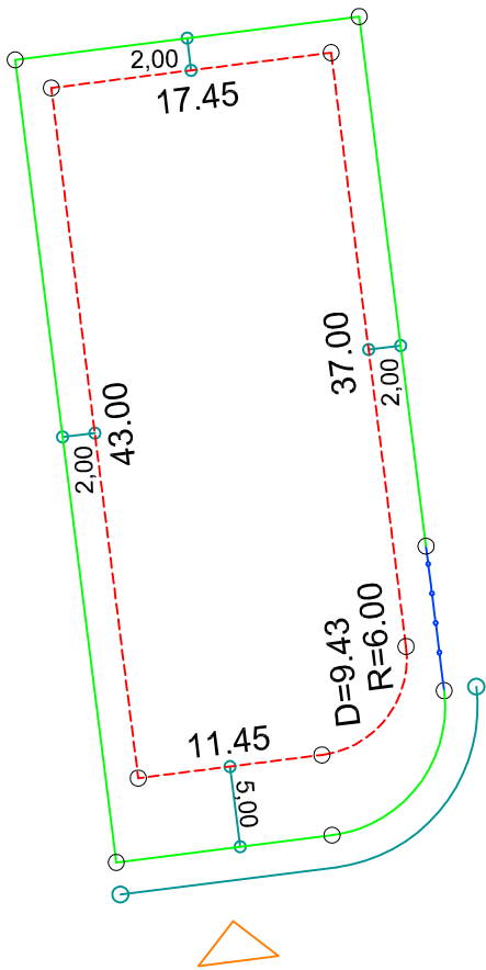
DETALHE DE RECUOS ESC.: 1/500
