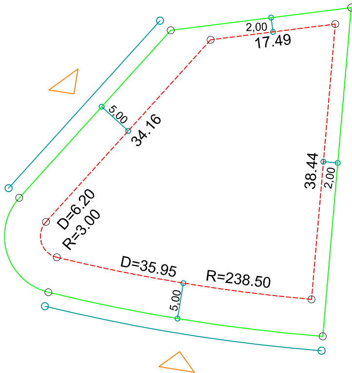
DETALHE DE RECUOS ESC.: 1/500
