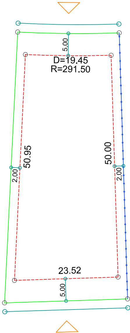
DETALHE DE RECUOS ESC.: 1/500
