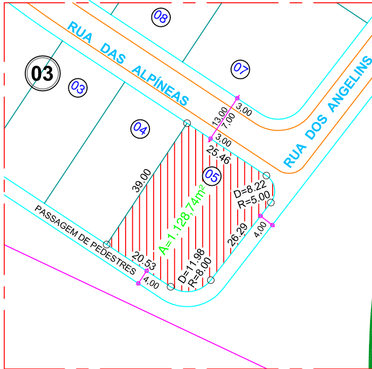
PLANTA DE SITUAÇÃO ESC.: 1/1000
