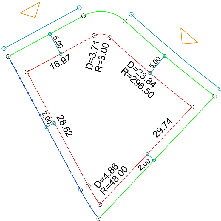
DETALHE DE RECUOS ESC.: 1/500
